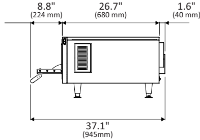
SEITENANSICHT MIT OFFENER TÜR
